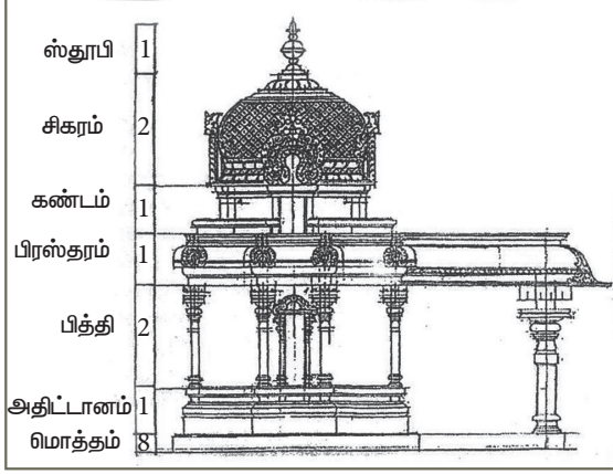
கோயில் விமானம்
